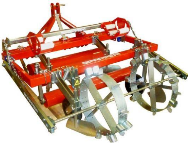
Dérouleuse et rouleau perforateur
